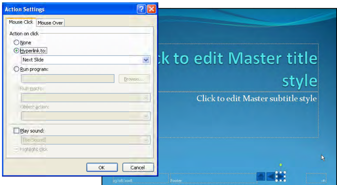
Hình 163. Tạo các nút Next và Previous
